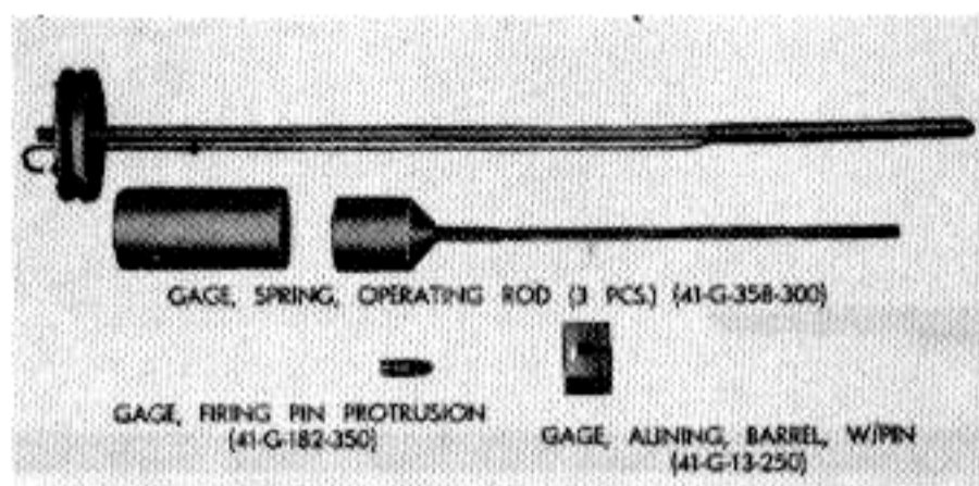
Fig. 99. Gages.
