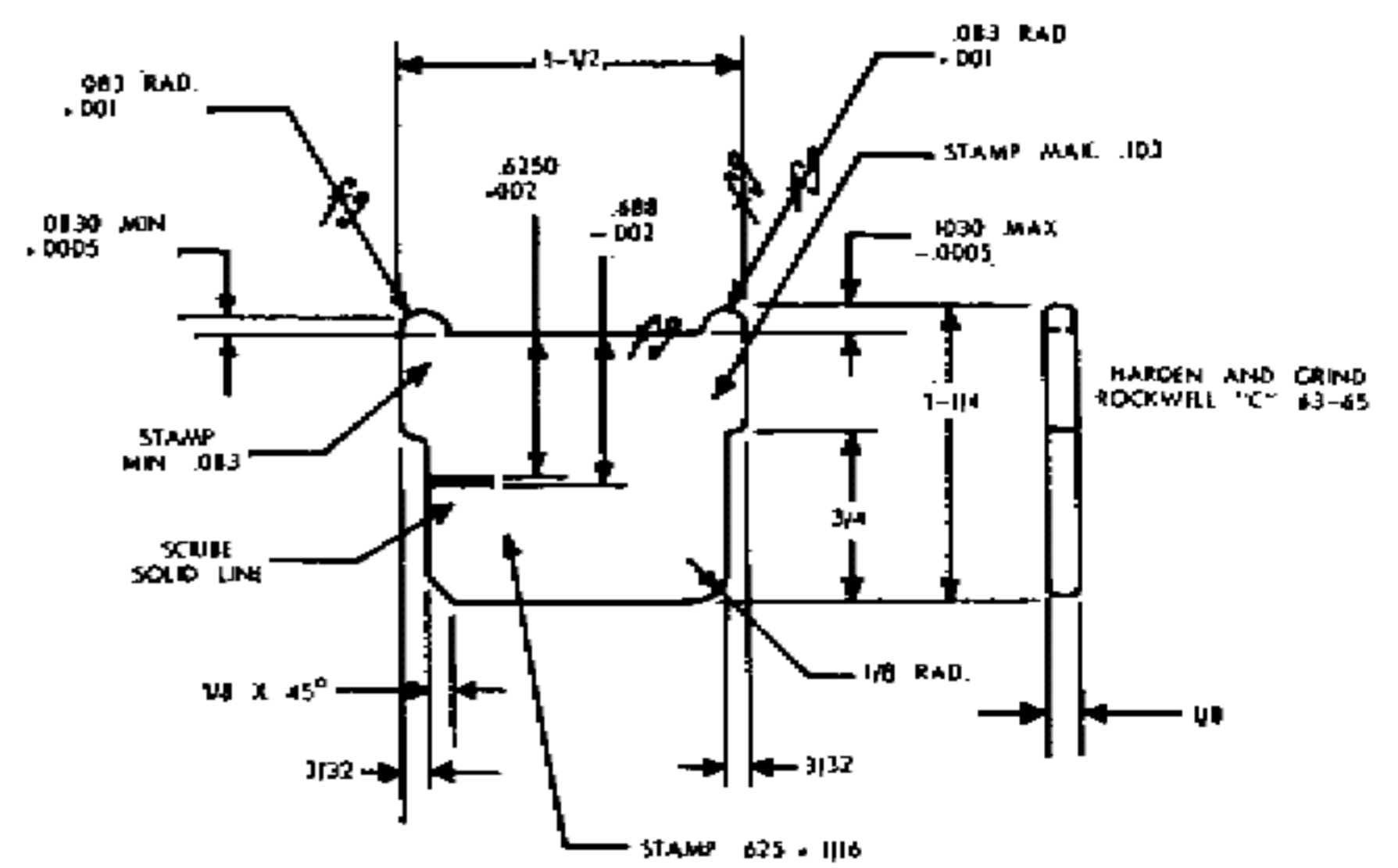
Fig. 110. Depth gage.
